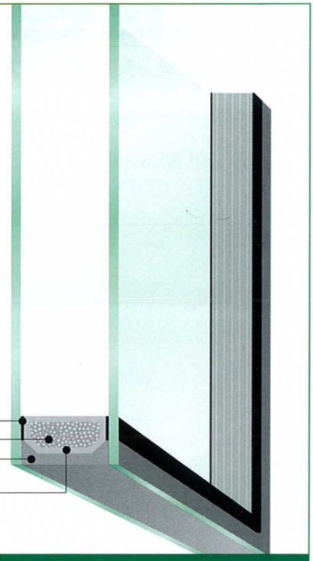
Schematischer Aufbau von Zweifach-Isolierglas
